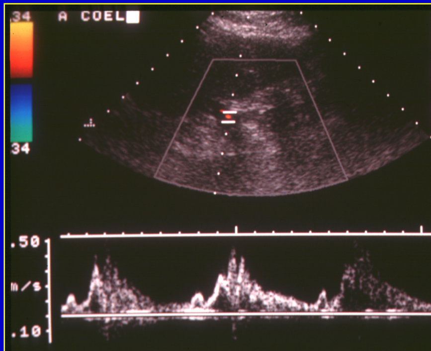
Tronc Coeliaque
